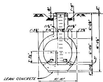
SECTION D-D
